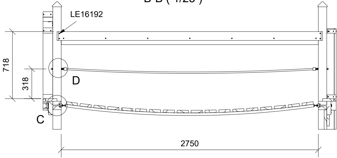
B-B ( 1/25 )
