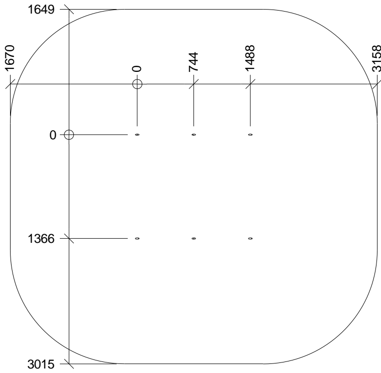
A-A ( 1/50 )
